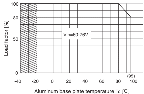
②Vin=DC60-76V
